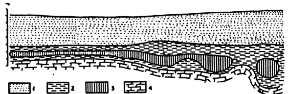
Ryc. 3. Przekrój przez złoża limonitów w Jasiowej Górze wg A. Białaczewskiego (1960).
